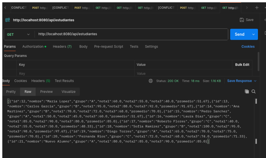
Figura 5: Petición GET en Postman
